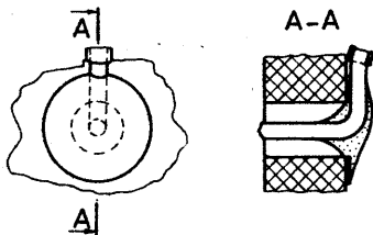
Obr. 9. Vodič na neosazeném pájecím bodě. Konec vodiče je viditelný na osazovací straně; příklad jednovrstvé desky s plošnými spoji s neprokovennými otvory
